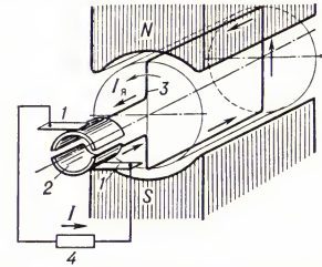
Рис. 1. Схема работы машины постоянного тока: N, S — полюса постоянного магнита; I — ток в нагрузке; 1 — щётки; 2 — пластина коллектора; 3 — виток провода на якоре машины; 4 — нагрузка.
